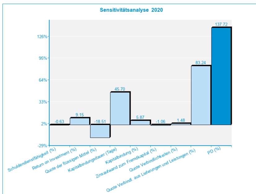
Abb. 6: Sensitivitätsanalyse II
