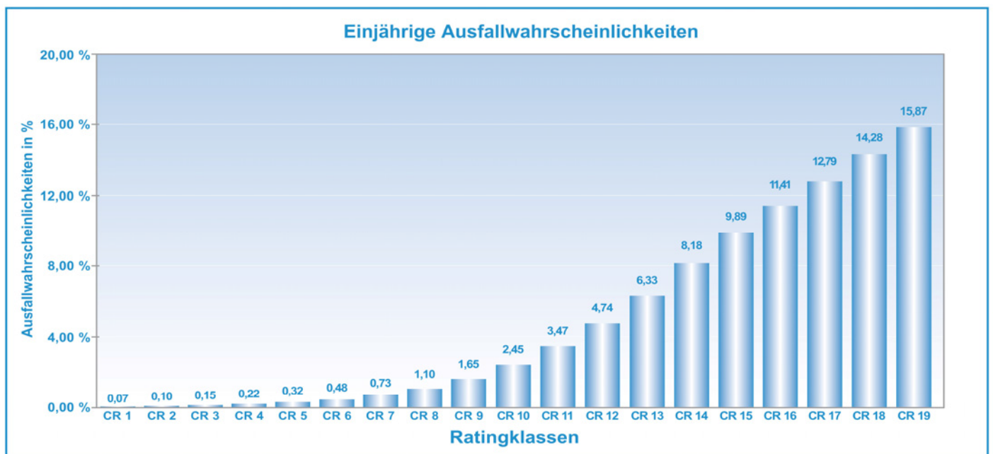
Abb. 4: Ausfallwahrscheinlichkeiten
