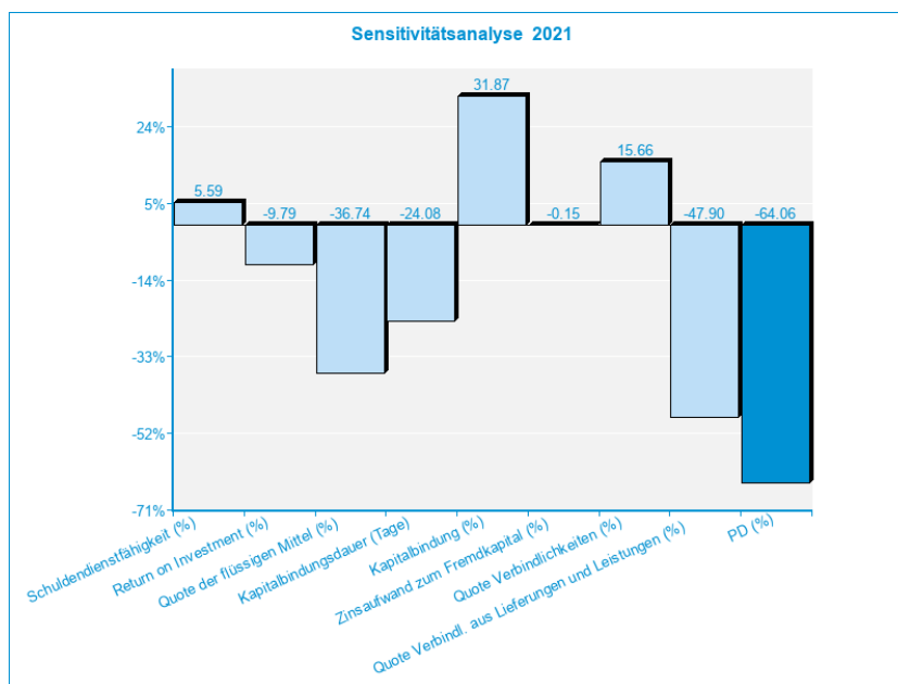
Abb. 5: Sensitivitätsanalyse I
